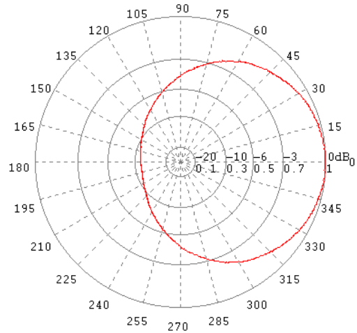
H-Ebene / H-Plane 230 MHz
